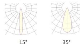
Valonjakokäyrät
